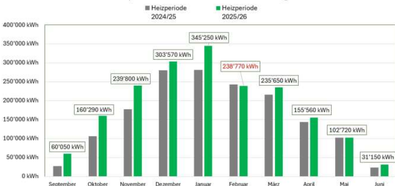
Fernwärmeproduktion im Jahres- / Perioden-Vergleich
